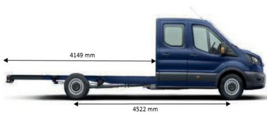
Chassis DC s dĺžkou L5
