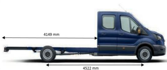
Chassis DC s dĺžkou L5
