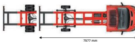
Chassis SC s dĺžkou L5
