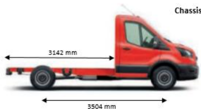
Chassis SC s dĺžkou L2
